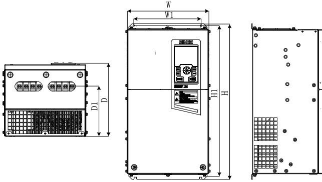
(c) 22kW~75kW 变频器外形
