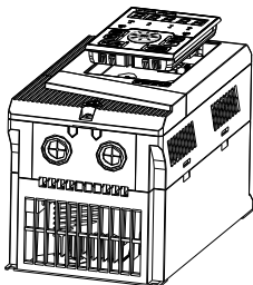
图 2-4 键盘安装图示
