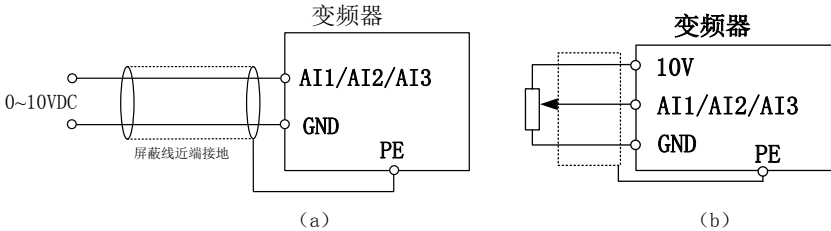
图 3-7 AI1、AI2、AI3 端子配线图
