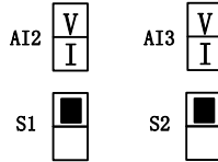
图 3-6 S4、S5 配置电压模式图
