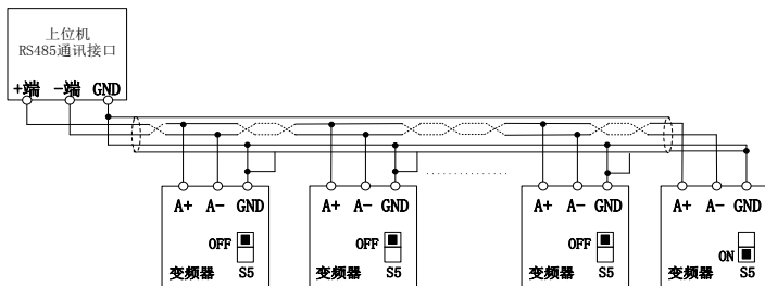
图 3-12 多台变频器通讯端子配线
