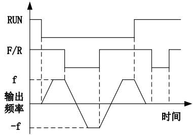
（b）F04.19=0，F00.03=0 运行正/反转逻辑
