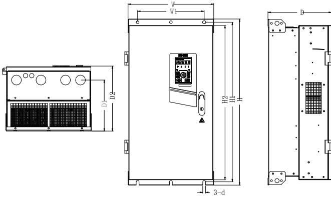
(d) 90kW~400kW 变频器外形
