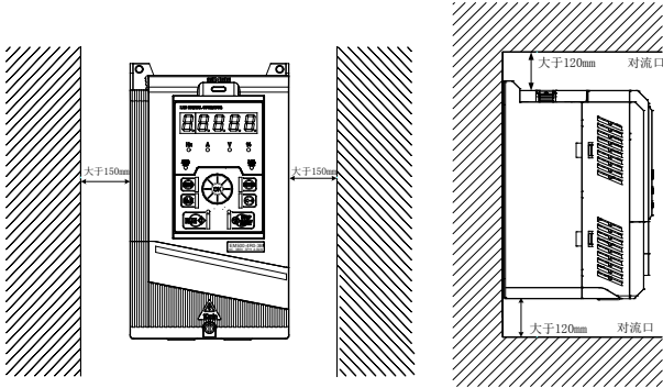
图 2-2 变频器安装方向和空间
