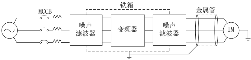
图 3-4 减少对外干扰的对策
