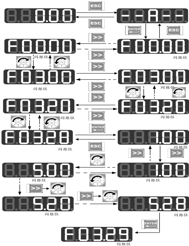
图 4-3 从上电至设置 F03.28=5.28 的操作流程图
