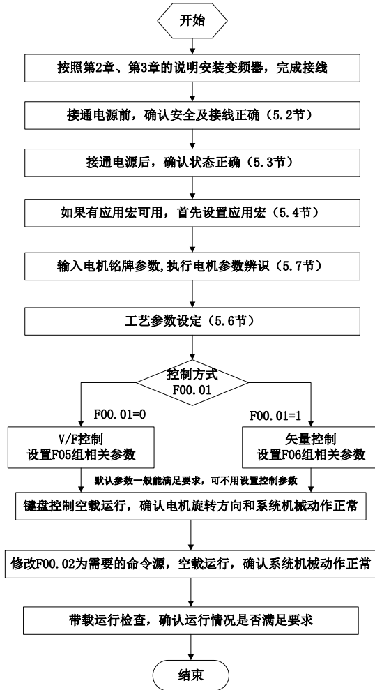
图 5-1 变频器调试流程图
