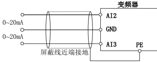
图 3-8 AI2、AI3 端子配线图
