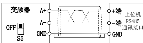
图 3-11 单台变频器通讯端子配线
