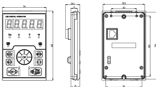
(a) 键盘尺寸
