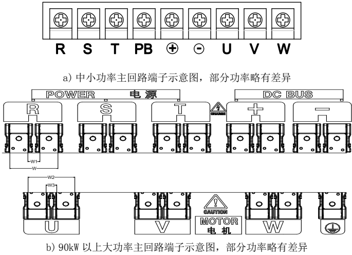
图 3-2 主回路端子排列示意图
