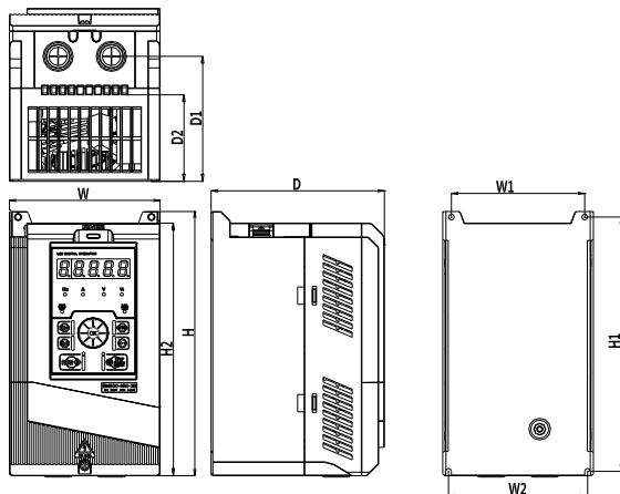
(b) 0.75kW~18kW 变频器外形
