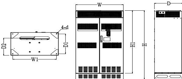
(e) 450~560kW 变频器外形
