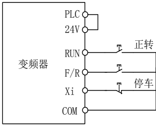
(a) F00.03=2 三线控制接线示意图 (b) F04.19=0，F00.03=2 正/反转运行逻辑
