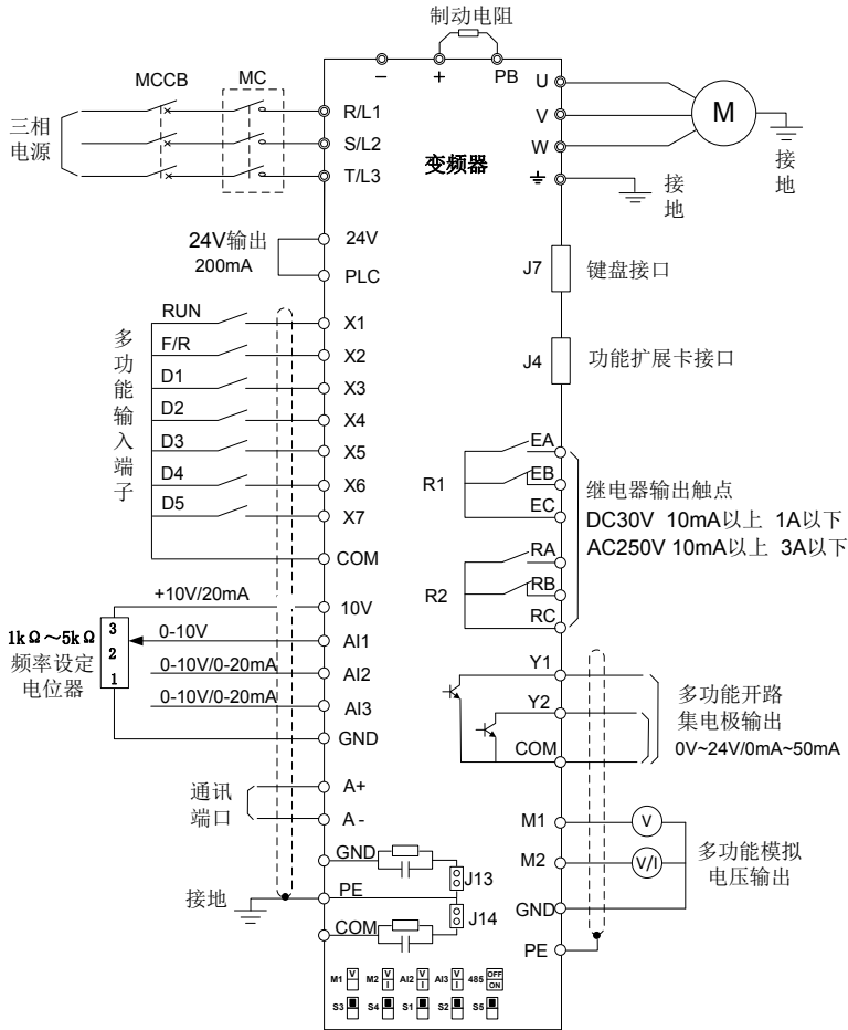
图 3-13 控制回路标准接线图
