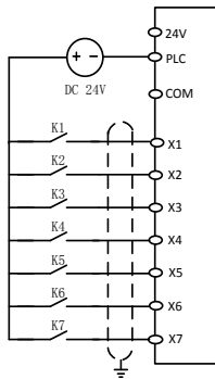
图 3-9 多功能输入端子接线图
